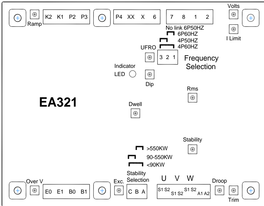
圖二 外型配置圖
